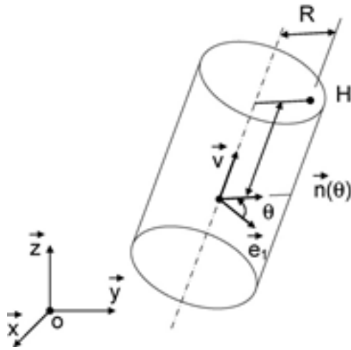
Fig. 9. Parametrizing a cylinder.
