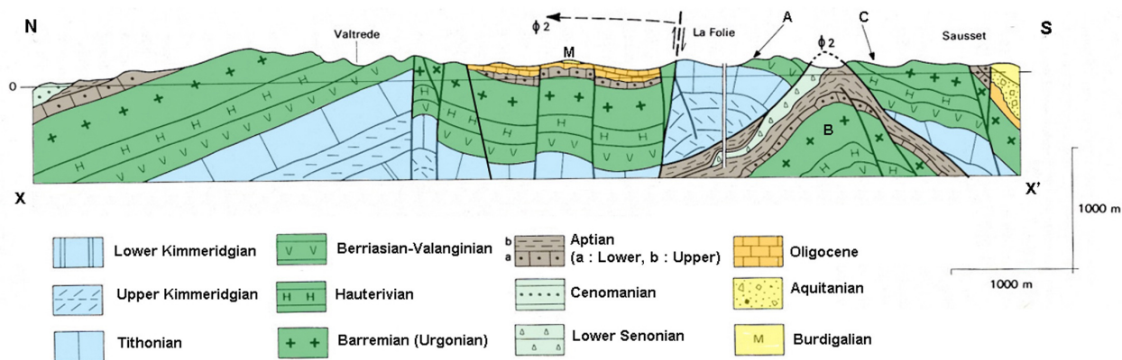
Fig. 3- Cross-section of La Nerthe range (after Guieu, 1977, modified). Location on Fig. 1 (section XX'). A. Chapats unit- B. La Folie-Valapaux faulted zone- C. Sausset unit. \Phi 2 : Southern La Nerthe overthrust. Fig. 3 Coupe du massif de La Nerthe (d'après Guieu, 1977, modifié). Localisation Fig. 1 (coupe XX'). A. Unité des Chapats- B. Zone faillée de La Folie-Valapaux- C. Unité de Sausset. \Phi 2 : chevauchement de la Nerthe méridionale
