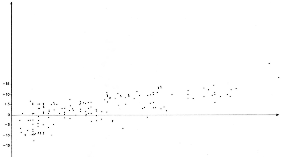
FIGURE 2a. - Altitude du toit de la grave (échelle horizontale : 1/2 000 e - échelle verticale : 1/500 e )
