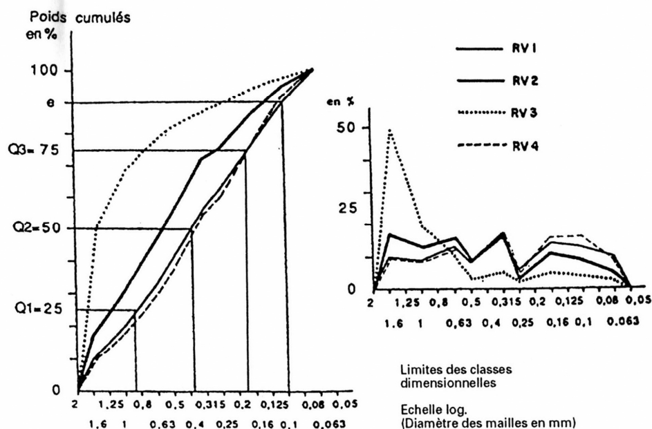
Fig. 3. – Courbes granulométriques cumulatives et simples des dépôts du ruisseau de Roque Vaoutade. RV 1: dépôt antérieur à l'incendie; RV 2: dépôt de l'automne 1989; RV 3: dépôt du printemps 1990; RV 4: dépôt du printemps 1991.
