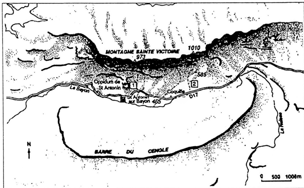
Fig. 1. – Croquis de localisation. 1: ruisseau des Deux-Aiguilles; 2: ruisseau de Roque Vaoutade.
