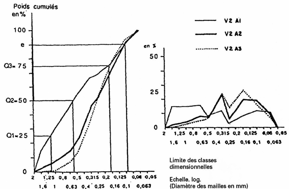
Fig. 2. - Courbes granulométriques cumulatives et simples des dépôts du ruisseau des Deux-Aiguilles. V2A 1: dépôt antérieur à l'incendie; V2A 2: dépôt de l'automne 1989; V2A 3: dépôt du printemps 1990.
