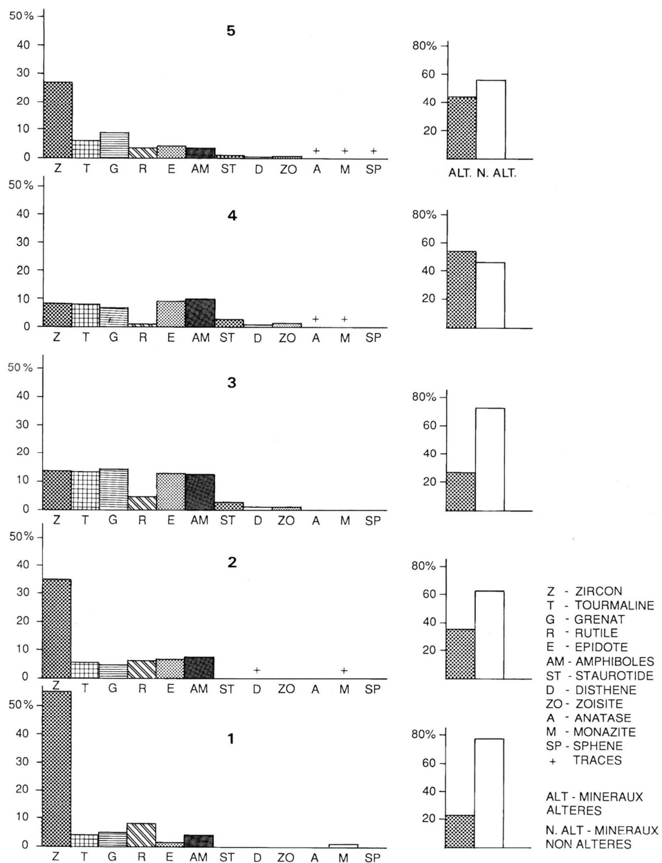
FIG. 6. - Minéraux lourds de la terrasse moyenne de l'oued makhrouga.
