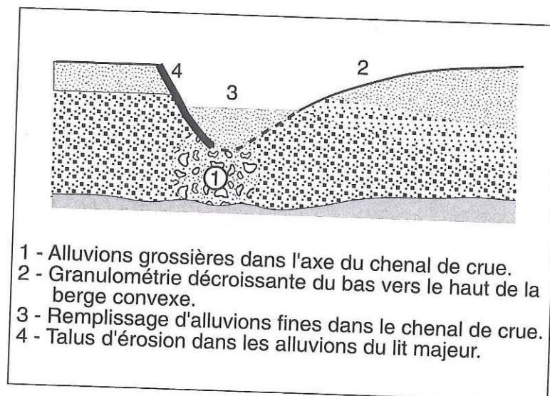
Figure 20 : Variations granulo- métriques types dans un lit moyen
