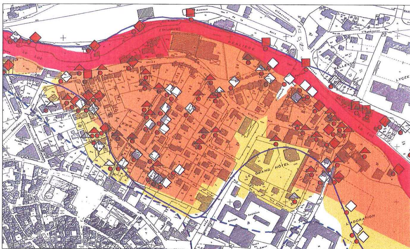
Figure 31 b : Mende (Lozère) - Cartographie : été 1994 - Inondation : septembre 1994
