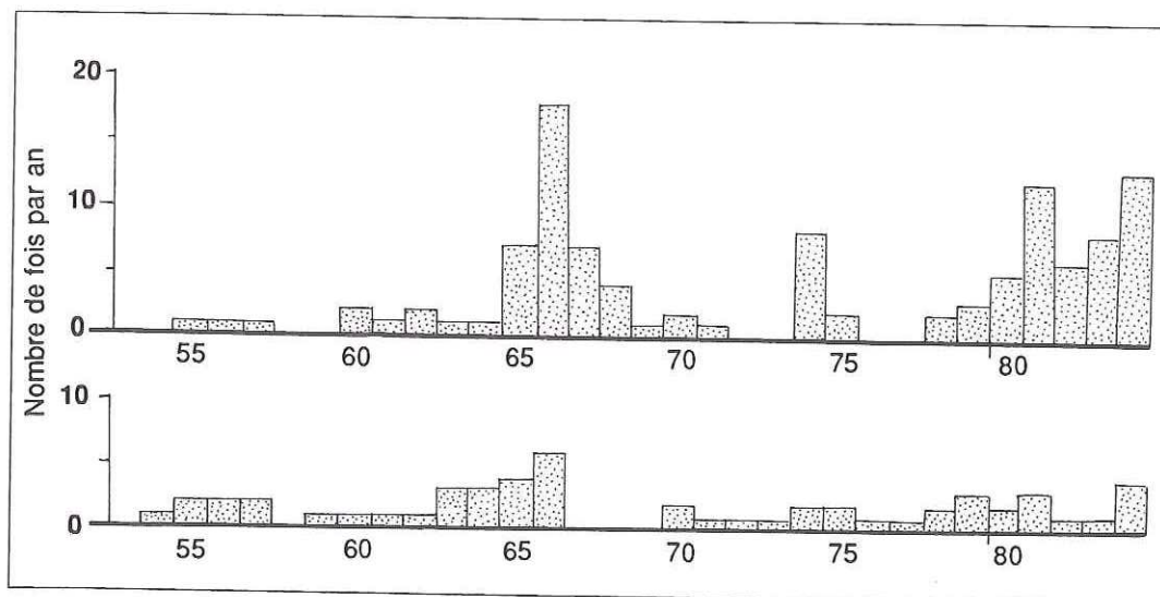
Figure 12 : Conséquences de la rectification du réseau hydrogra- phique du Ger (Belgique) sur la périodicité des crues (d'après G. Mabilie et F. Petit, 1987). Le premier gra- phique indique le nombre de fois où les débits ont été égaux ou supérieurs à 5 m 3 /s. Le second graphique indique le nombre de fois où, en une année, se sont pré- sentées des périodes de 3 jours consé- cutifs où plus de 40 mm de pluie ont été recueillis. N.B : la rectification du réseau du Ger a été achevée en 1980.
