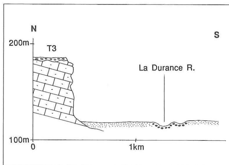
Figure 9 : La terrasse T3 (Pléistocène moyen ?) de la Durance tronquant la molasse à Lauris (Vaucluse)
