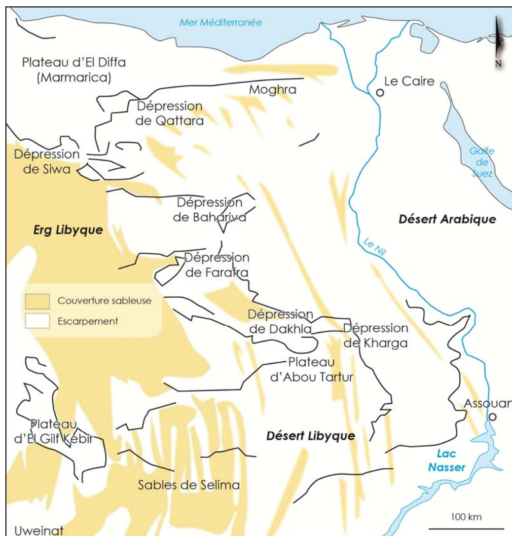
Figure 14 - Répartition des couvertures sableuses dans le désert libyque.
