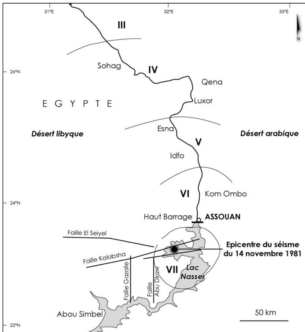
Figure 7 - Répartition de l'intensité sismique le 14 novembre 1981.
