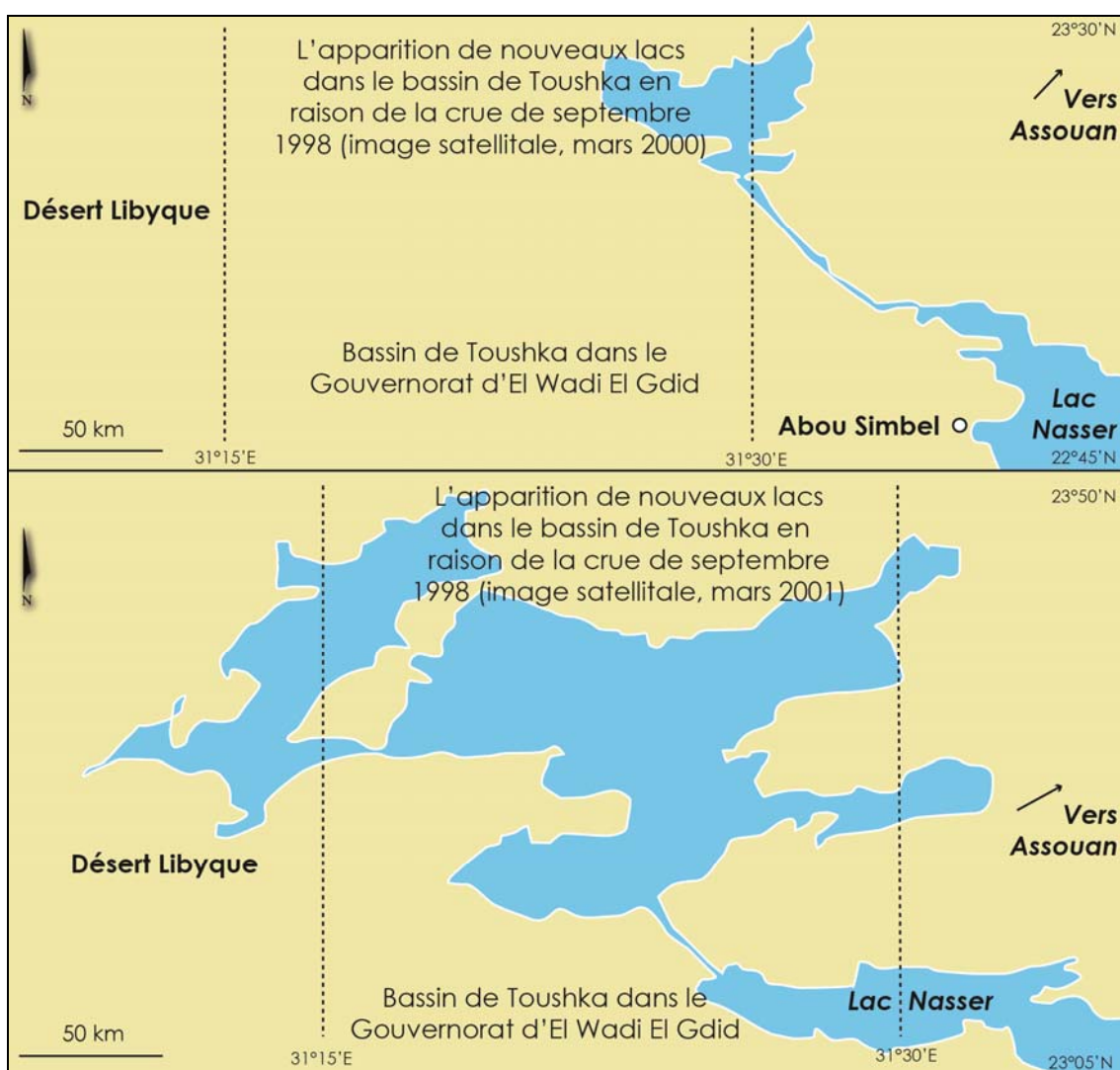
Figure 13 - Apparition de nouveaux lacs dans le bassin de Tushka après la crue de 1998.
