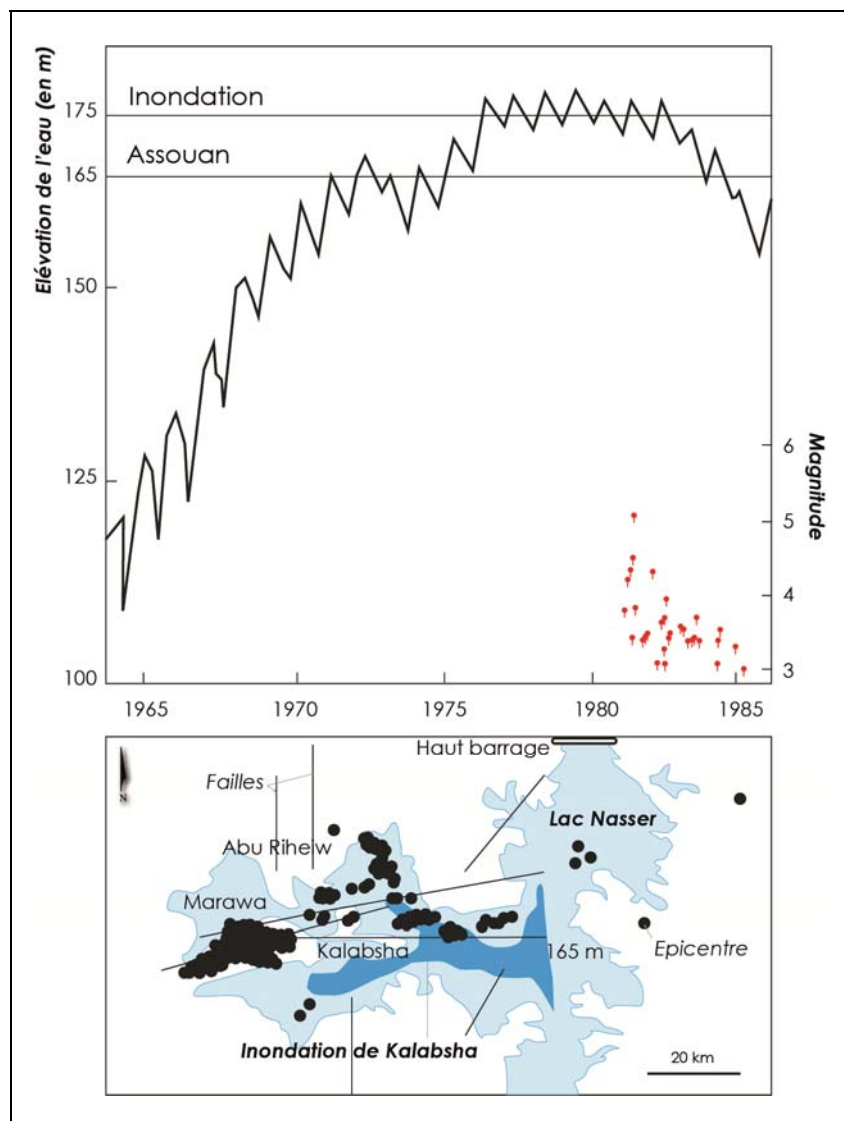
Figure 10 - Élévation du niveau de l'eau dans le lac Nasser (1964-1986) et tremblements de terre les plus importants après l'inondation des zones de Kalabsha et Marawa.
