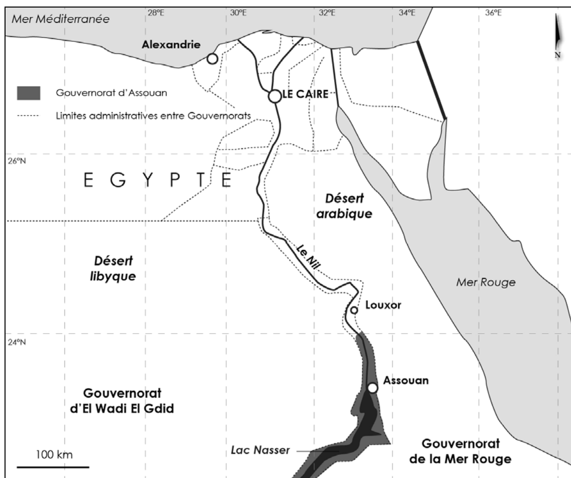
Figure 1 - Carte de localisation du gouvernorat d'Assouan.
