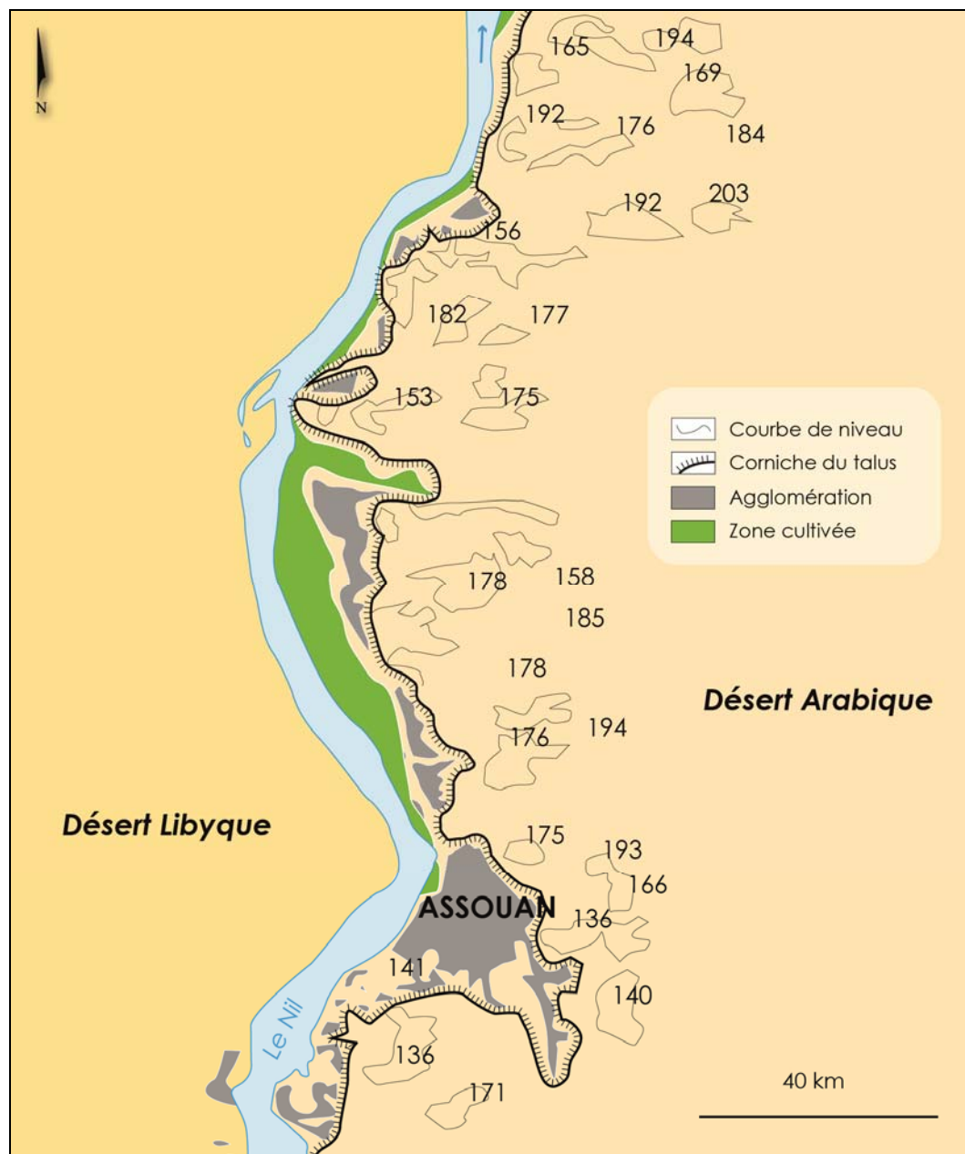
Figure 5 - Carte de localisation du phénomène de chute de blocs.
