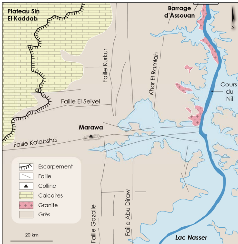
Figure 9 - Carte géologique de la partie occidentale du lac Nasser.
