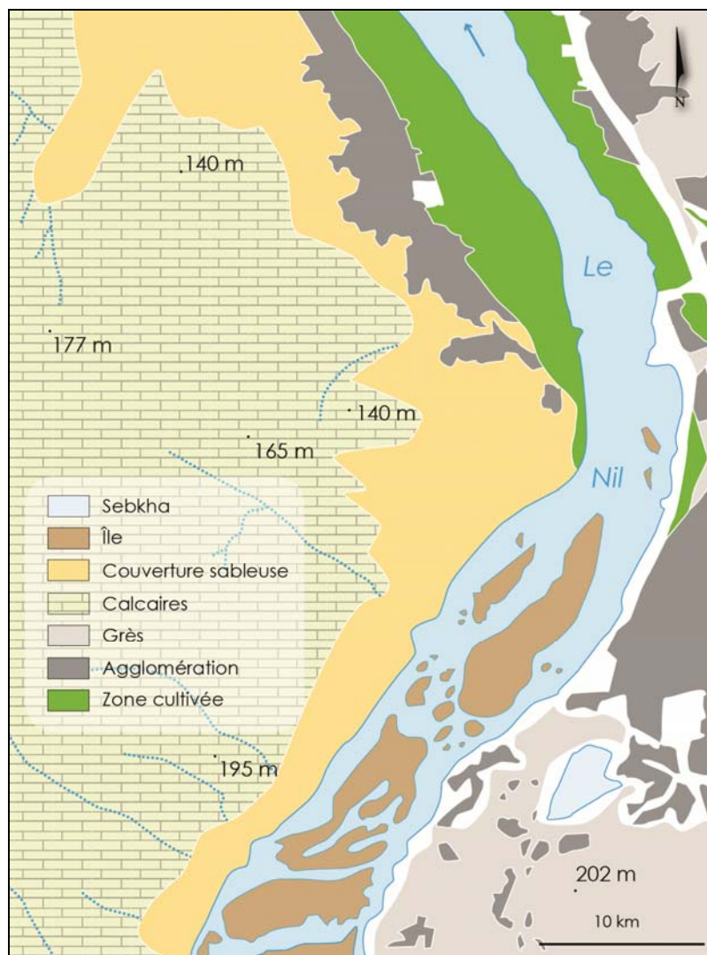
Figure 15 - Carte des formations éoliennes et localisation des zones exposées au risque d'ensablement à Assouan.
