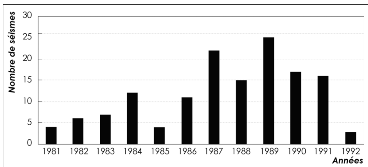
Figure 11 - Nombre de séismes à Assouan entre 1981 et 1992.
