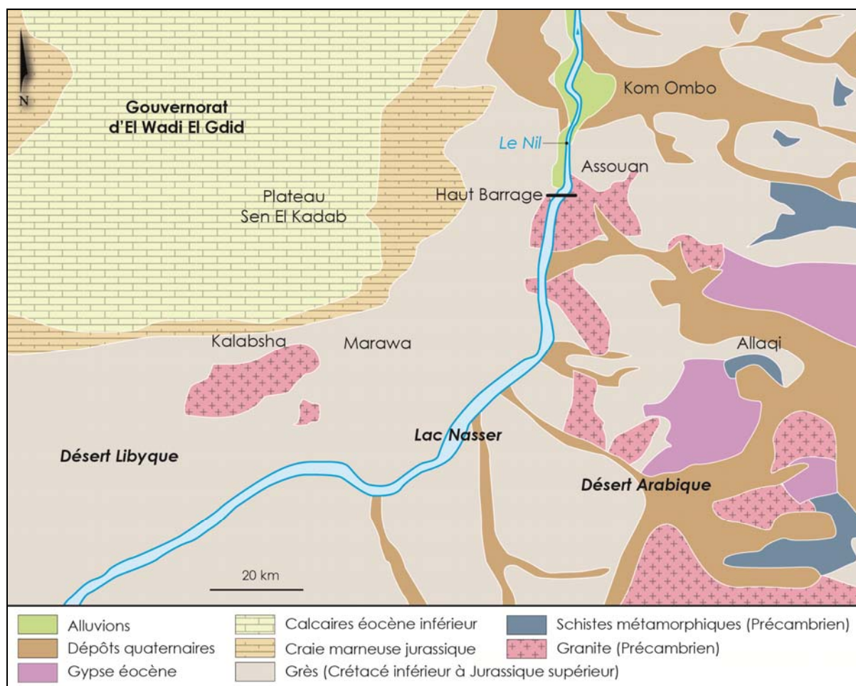
Figure 2 - Carte géologique simplifiée du gouvernorat d'Assouan.
