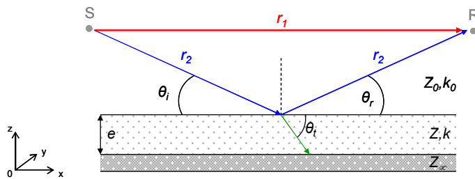
Figure 23. Représentation schématisée de la configuration géométrique étudiée : Trajets des ondes directe ( r_1 en rouge) et réfléchi ( r_2 en bleu) de la source au récepteur, au-dessus d'un sol parfaitement plan et partiellement réfléchissant (matériau bicouche)
