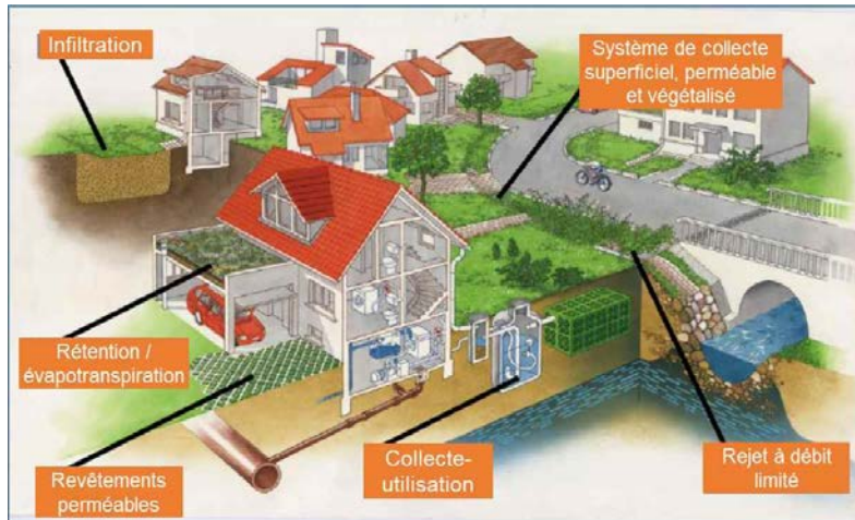
Figure 13. Gestion naturelle des eaux pluviales, adapté de Bayerisches Landesamt für Umwelt « Naturnaher Umgang mit Regenwasser »
