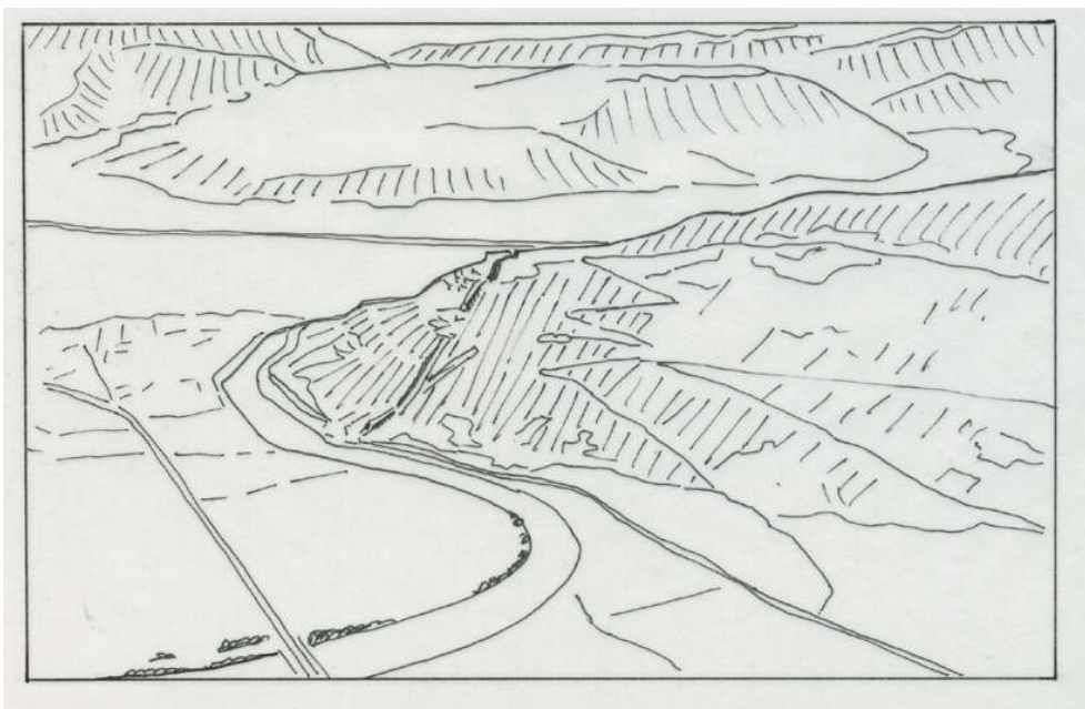
Figure 4 : Croquis de l'auteur d'après une image d'écran oblique-3D de l'espace correspondant à l'aquarelle Alpine landscape vu de l'E: la vallée de l'Isère, le versant est du Mont Rachais et la clue de Grenoble à l'arrière-plan
