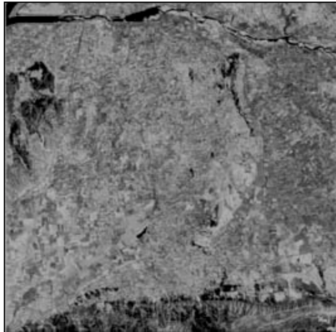
Figure 3 : Image satellitale (Landsat 5 TM).
