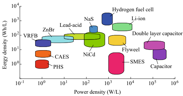
Fig. 4 Ragone chart
