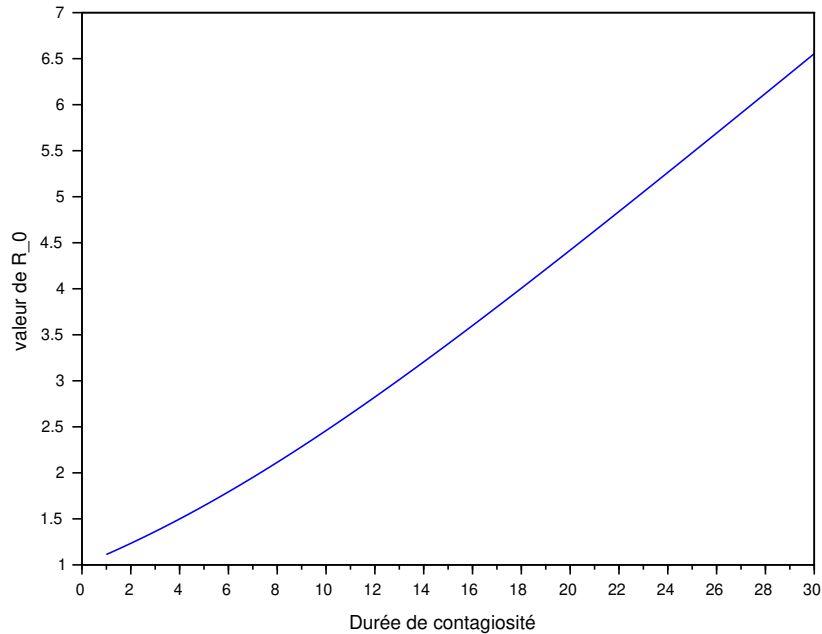
Lien entre R_0 et la durée de contagiosité T_c pour \lambda = 0.218
