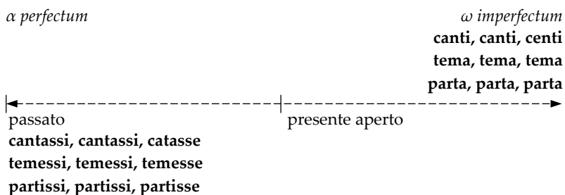
Fig. 61: Modo congiuntivo ossia Cronotesi in fieri
