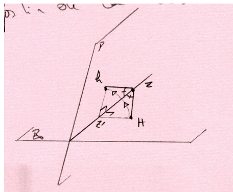
FIGURE 14 – Angles et distances préservés par le rabattement.
