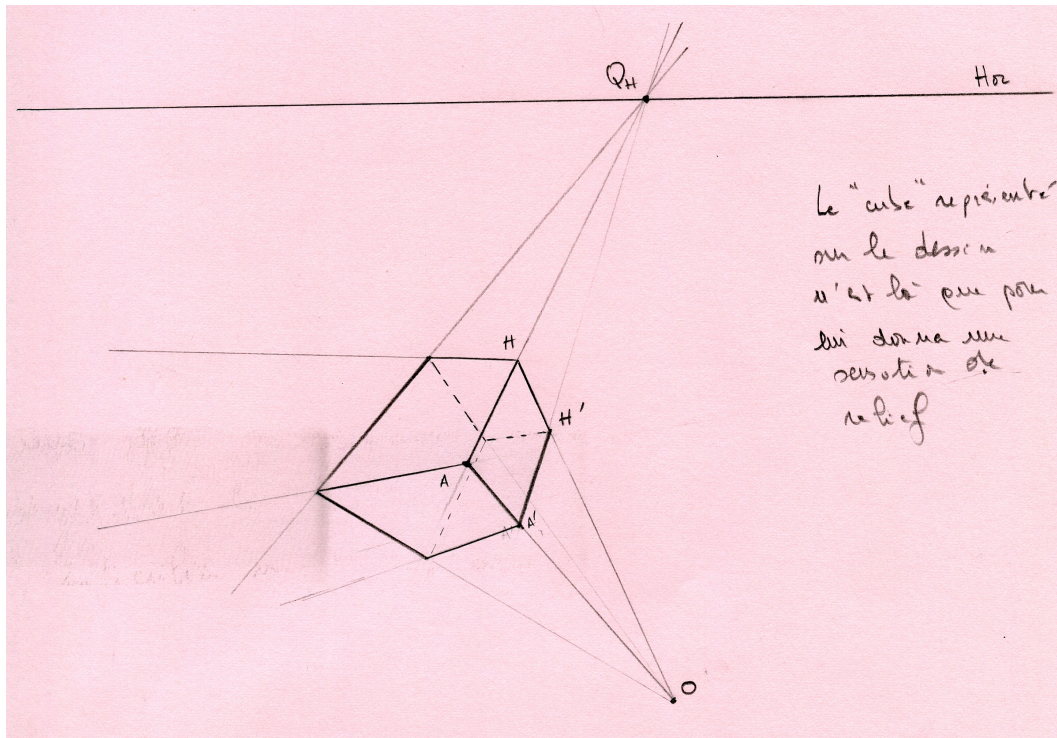
FIGURE 9 – Construction de points en surplomb.
