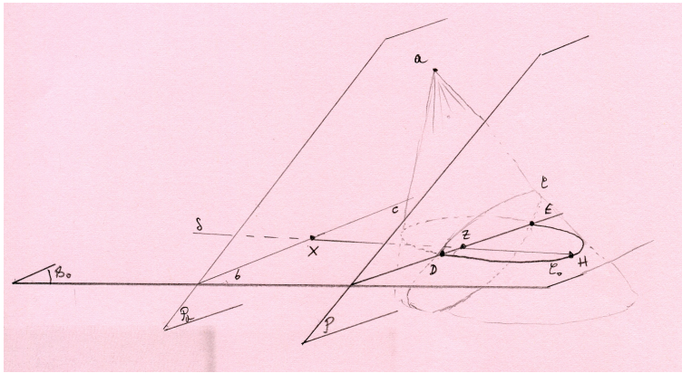
FIGURE 13 – La génération de la Hire : générer une conique à partir d'un cercle.
