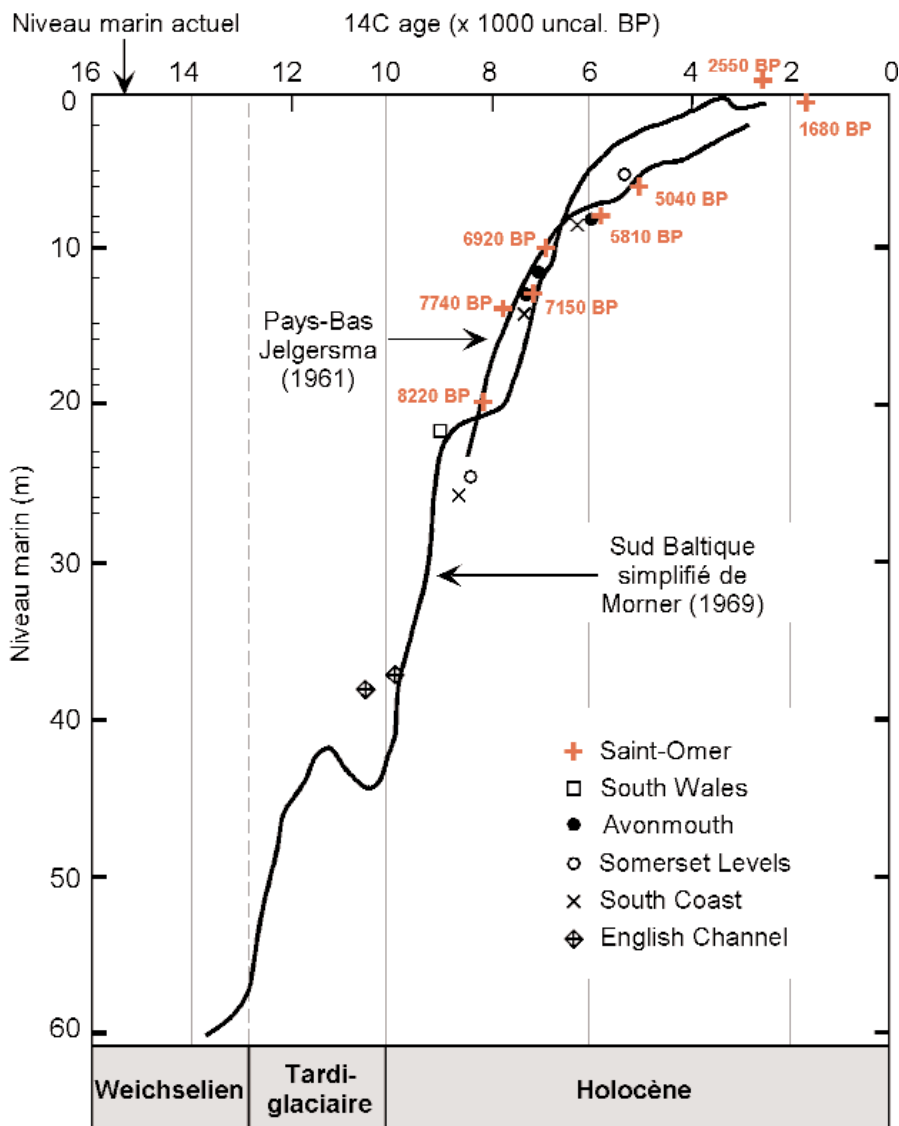
Fig. 11 - Remontée du niveau marin lors de la transgression tardiglaciaire/holocène (d'après Jelgersma, 1961 ; Mörner, 1969 ; in Hutchinson, 1992). Les dates radiocarbonees sont non calibrées.
