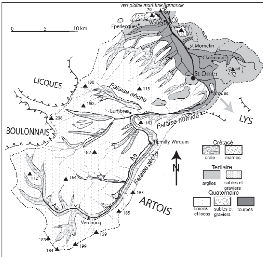
Fig. 2 - Lithologie du bassin versant de l'Aa et du bassin de Saint-Omer, depuis Verchocq jusqu'à Watten. La flèche grise représente l'ancienne vidange (jusqu'au Quaternaire ancien) de l'Aa dans le bassin de la Lys.
