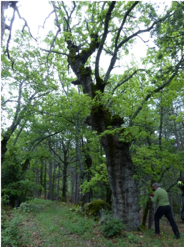
Figure 6 : Carottage d'un chêne (Chastranelle, Courbons, Digne-les-Bains) afin de construire un référentiel local pour cette essence.
