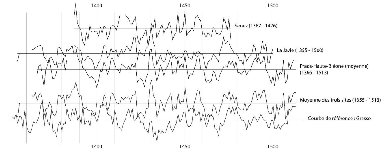
Figure 5 : Position de synchronisation des séries dendrochronologiques des trois sites (séries standardisées par la méthode du Corridor de G.-N. Lambert). Dans la partie inférieure du graphique, la moyenne de ces trois sites corrèle avec la chronologie de référence de la ville de Grasse (établie par S. Wicha, société Archéobois)
