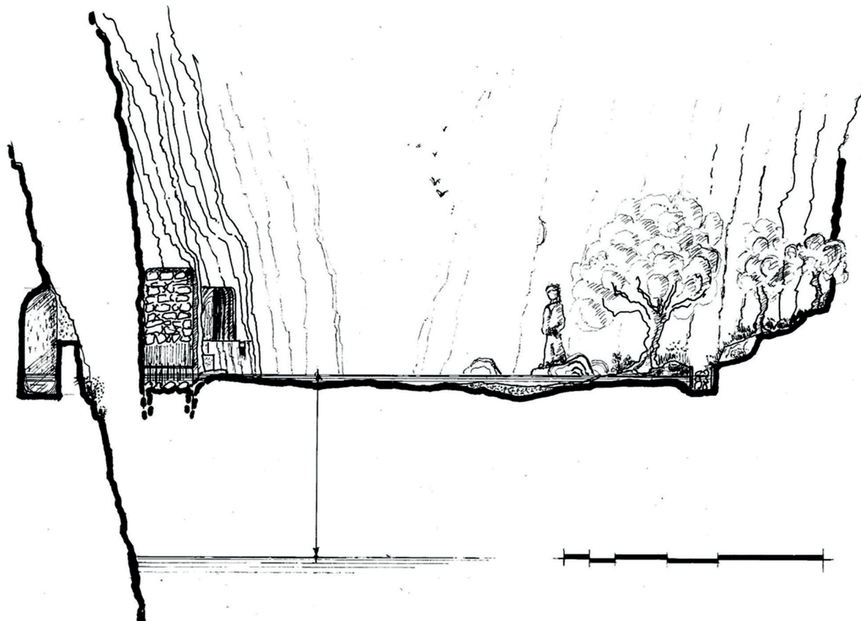
Fig. 19 – Restitution du barrage de la Bottigliera (© Ph. Lenhardt- J.-L. Paillet, Mission HydroSyra).
