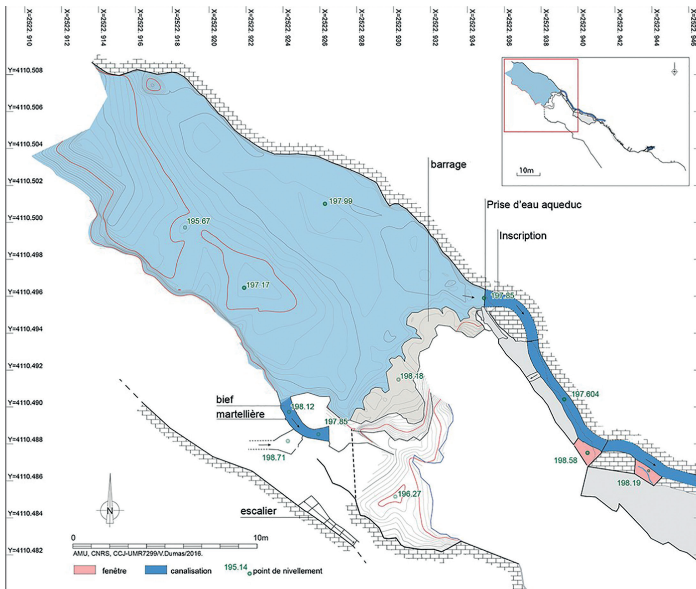
Fig. 17 – Le captage de la Bottigliera (© V.Dumas, Mission HydroSyra).
