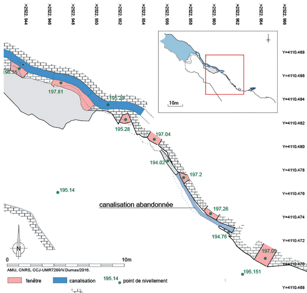
Fig. 10 – Planimétrie de la modification du tracé, Bottiglieria (© Plan V.Dumas, Mission HydroSyra).
