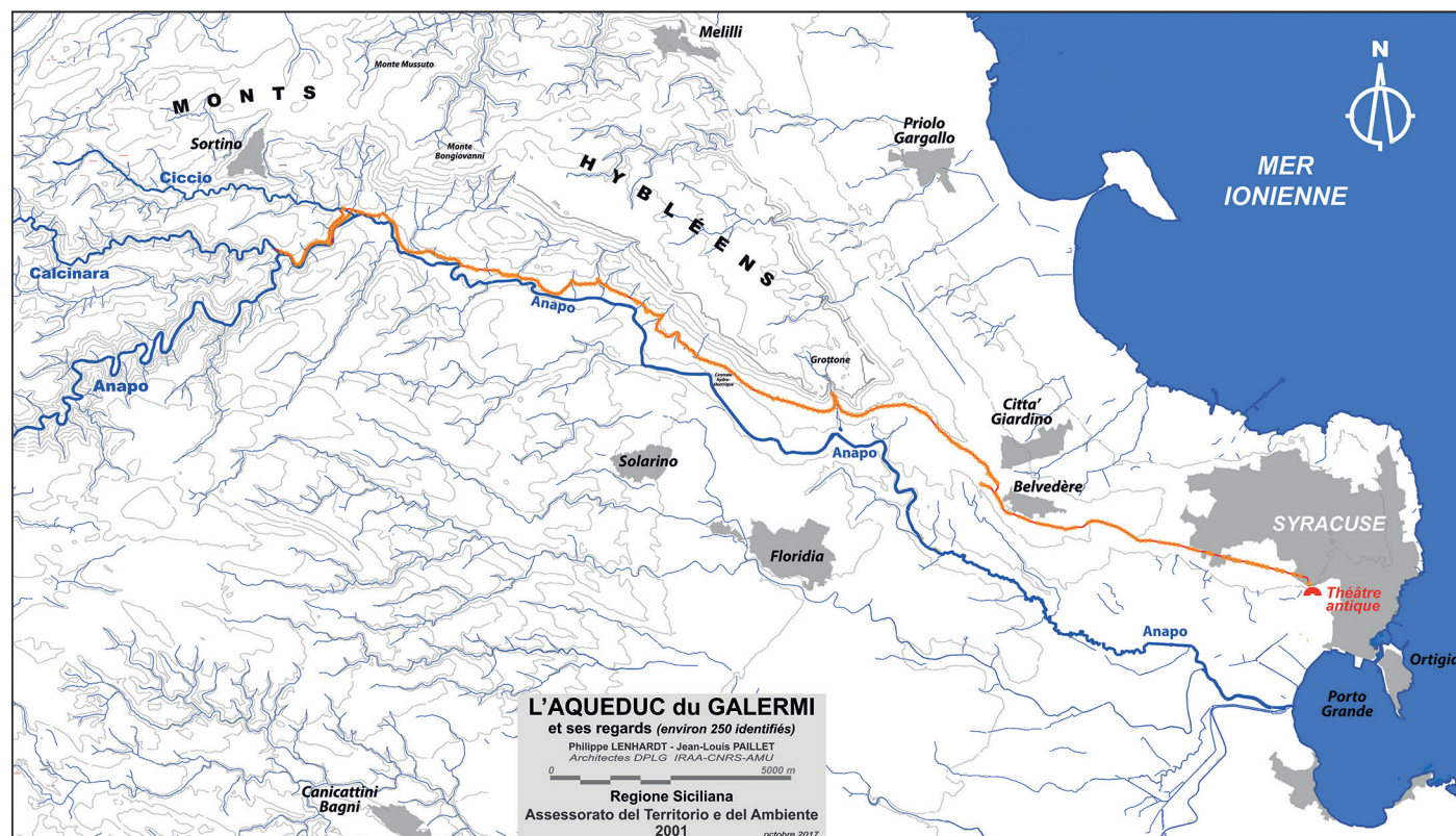
Fig. 1 – Tracé général de l'aqueduc (© Ph.Lenhardt, J.-L.Paillet, Mission HydroSyr).
