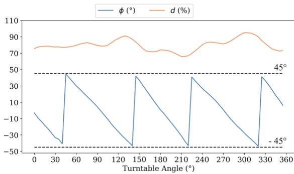
Figure 9. Mesure de l'orientation (cap) du plateau tournant réalisées par la méthode des moindres carrés décrite dans [5] comparée à l'orientation réelle du plateau tournant.
