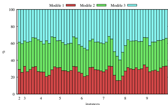
FIGURE 7 – Rapport en pourcentage du temps consommé par chaque modèle sur le temps cumulé des modèles \mathcal{M}_{i_1} , \mathcal{M}_{i_2} et \mathcal{M}_{i_3} en fonction des instances classées selon le nombre n d’hexagones souhaités.
