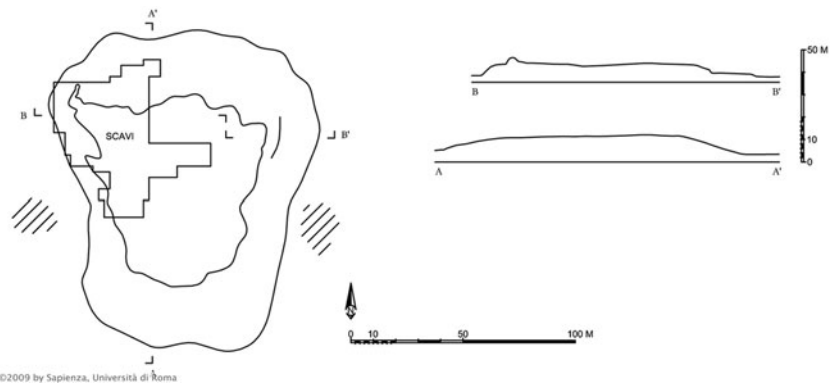
Figure 5. Uch Khulakh: plan of a single tepe. (© Università degli Studi di Roma; Silvi-Antonini & Mirzaakhmedov 2009.)
