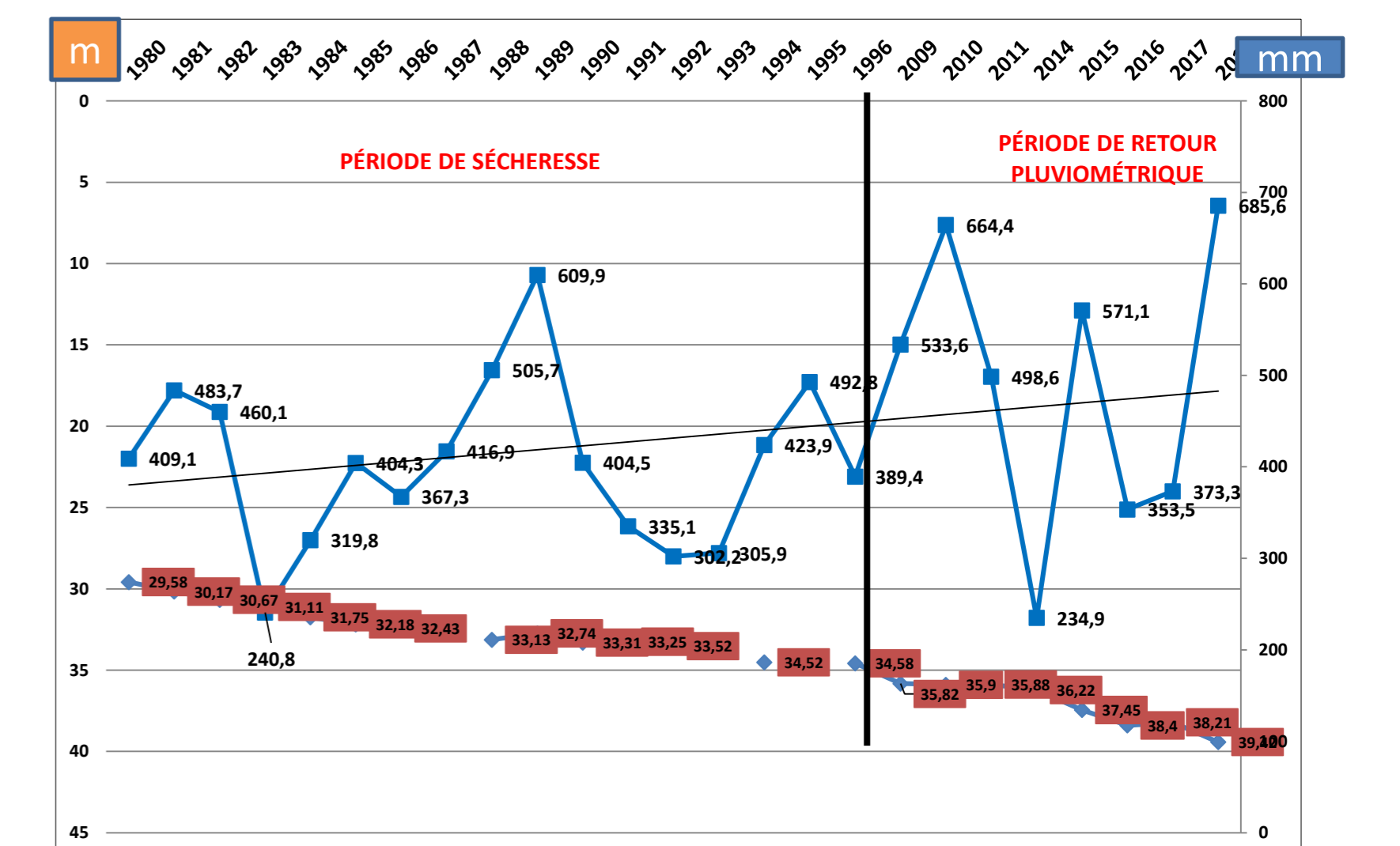
Figure 1: Suivi des variations pluviométriques et des niveaux statiques (NS) de la Nappe du Continental Terminal (CT)
