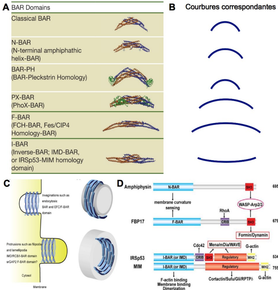
Figure 6: Classement des différents domaines BAR et de leurs effet sur la membrane.(A) Table des différentes protéines contenant les différents types de domaines BAR.(B) Présentation des différentes courbures correspondantes aux types de domaines présentés en (A).(C) Exemple d'utilisation des domaines BAR lors de l'endocytose et de la formation de filopodes.(D) Organisation modulaire des différents domaines BAR. Les domaines BAR font toujours parti de protéines multi-domaines et en particulier des domaines de régulation de l'actine, de liaison au protéine de régulation, de domaine d'activation et de signalment. Ainsi de nombreux domaines BAR ont des domaines de recrutement pour certaines membranes ou protéines d'échafaudages (SH3). Certain domaines BAR présentent les site de recrutement des GTPases (activation/inhibition) (CRIB), ainsi que des domaines de liaisons à l'actine monomérique (WH2).
