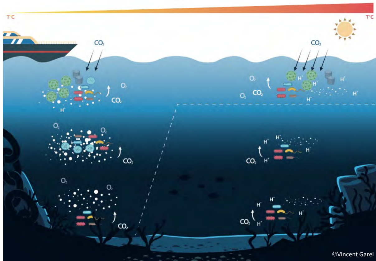
Figure 1-5 Infographie représentant de manière schématisée les impacts du changement climatique sur les zones méso- et bathypélagique. L'augmentation de la température de surface augmente la stratification des eaux de surface, limitant les échanges avec les eaux sous-jacentes. Par conséquent, le CO 2 s'accumulerait en surface provoquant l'acidification des eaux de surfaces. La matière organique produite en surface est principalement consommée par les communautés de surfaces ce qui diminue l'export vers les zones méso- et bathypélagique, donc diminuerait la séquestration du carbone. Enfin, le front thermique diminuerait la diffusion de l'oxygène vers les zones plus profondes modifiant la ventilation des eaux profondes (accroissement des zones à minimum d'oxygènes – OMZ). La ligne en pointillé représente la stratification des eaux. Illustration réalisée par Vincent Garel.
