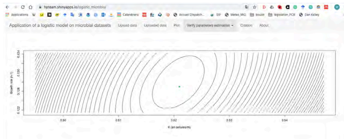
Figure 6-5 Représentation en contour-plot 2D de la minimisation de la somme résiduelles des carrés. Le point vert représente les coordonnées des paramètres estimés ( \mu_{\max} et K )
