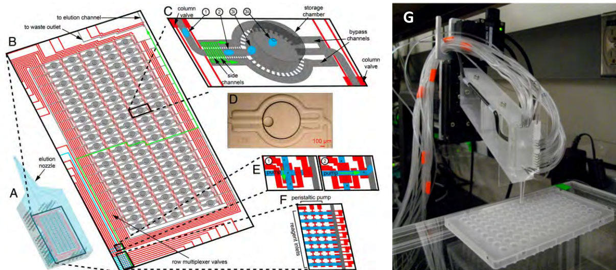
Figure 5-2 Réseau de réacteurs microfluidiques programmables tiré de l'article de Leung et al. (2012) . Les légendes des schéma A, B, C, D, E, F sont une traduction de la légende originale. (A) Schéma du dispositif montrant la structure d'une buse d'éluion conçue pour s'interfacier avec des tubes microfuges standards pendant l'éluion des chambres. (B) Réseau adressable de 95 chambres de stockage organisées en 19 rangées et 5 colonnes. Les couches de contrôle sont indiquées en rouge. L'actionnement du multiplexeur de rangées et des vannes de colonnes crée un chemin fluide unique (flèche verte) s'écoulant des ports de haute et de basse pression. (C) Géométrie de l'élément de stockage pour l'immobilisation et la coalescence des gouttelettes contrôlées par le flux. (1) Pendant le transport vers un élément de stockage adressé, un mince film d'huile lubrifiant empêche le mouillage des parois des canaux. (2) Les canaux latéraux créent une dérivation pour l'huile (flèches vertes), réduisant la vitesse des gouttelettes. (3i) En dessous de la vitesse d'écoulement critique, la gouttelette entre dans la chambre et se positionne à l'extrémité de la chambre cylindrique. (3ii) Au-dessus de la vitesse d'écoulement critique, la gouttelette ne se positionnent pas à l'entrée mais se déplace dans la chambre et s'immobilise au plafond de la chambre. (D) Micrographie d'une gouttelette d'eau stockée de 2,7 nL. (E) Module de triage des cellules. (1) Une suspension monocellulaire est pompée dans le canal de triage. (2) La cellule est encapsulée dans une gouttelette pour être transportée vers l'arrière de la chambre. (F) Module de dosage des réactifs. G Photographie d'une buse d'éluion montée sur un bras articulé 3 axes.
