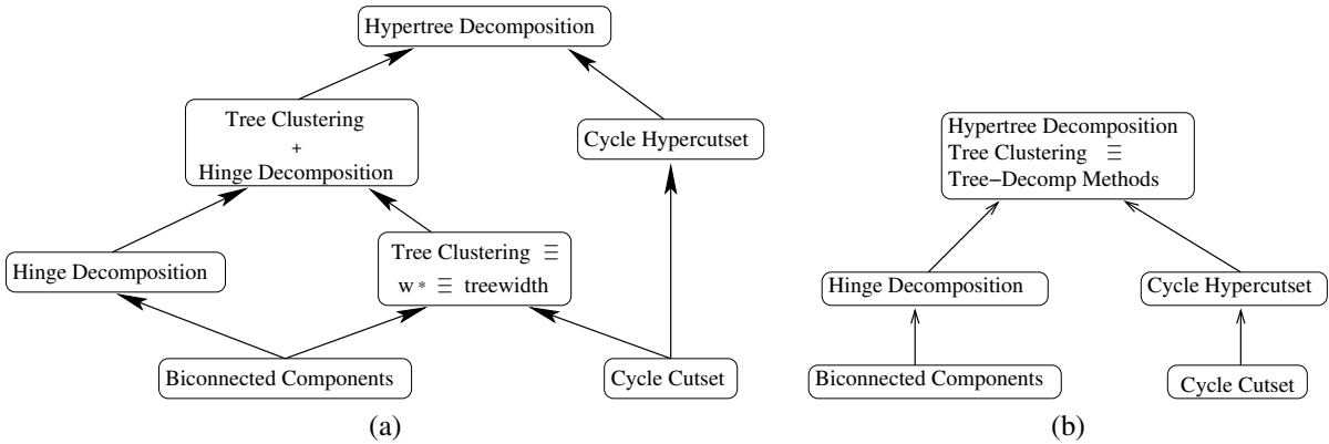
FIGURE 3.1 – (a) La hiérarchie des méthodes de décompositions structurelles (Gottlob et al., 2000), (b) la hiérarchie mise à jour grâce à la nouvelle évaluation de la complexité de nFC_{2m} .
