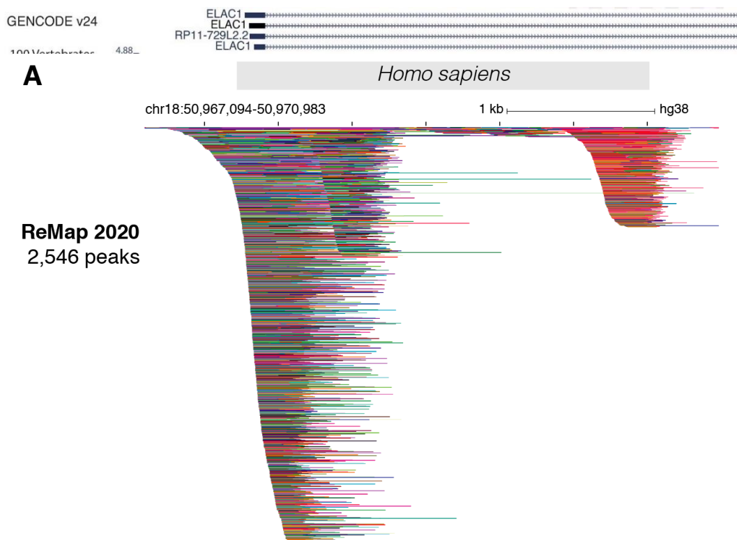
Figure I.2 : Visualisation des données de fixation des protéines régulatrices de ReMap au niveau d'une région promotrice chez l'Homme.
