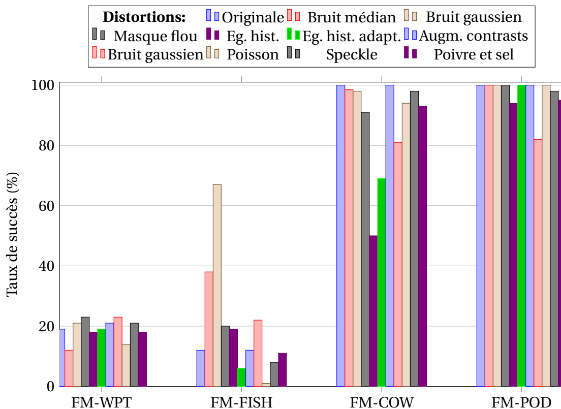
FIGURE 1.14. – Taux de succès de l’autofocus (abscisse), selon la mesure de focalisation utilisée (ordonnée) et de la distorsion appliquée (couleurs), sur des cas classiques d’utilisation (contrastes standards).
