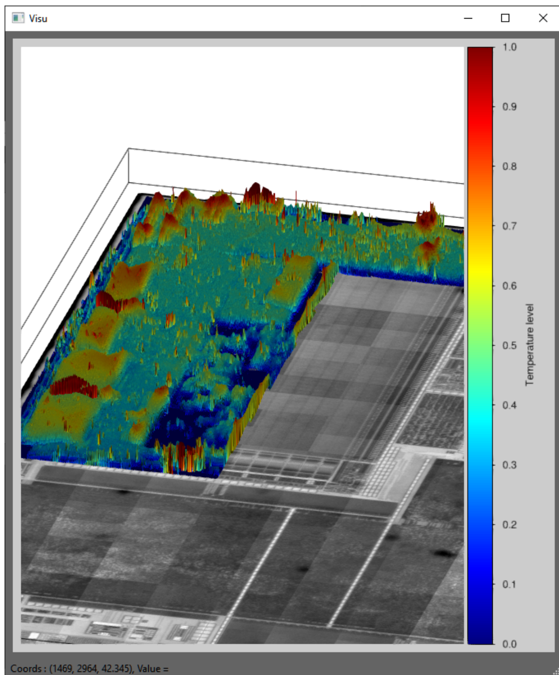
FIGURE 3.10. – Affichage 3D de l’image d’un composant et de données relatives à sa caractérisation de zones d’intérêt (ici la température).
