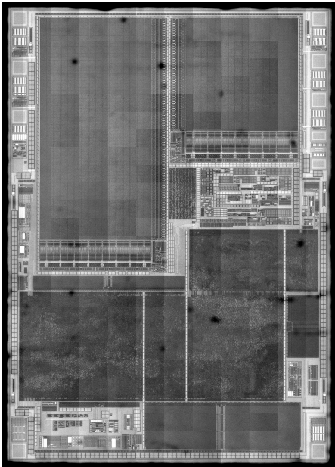
FIGURE 3.3. – Résultat de l'assemblage des imagerie acquises lors du balayage d'un circuit électronique au 20x.
