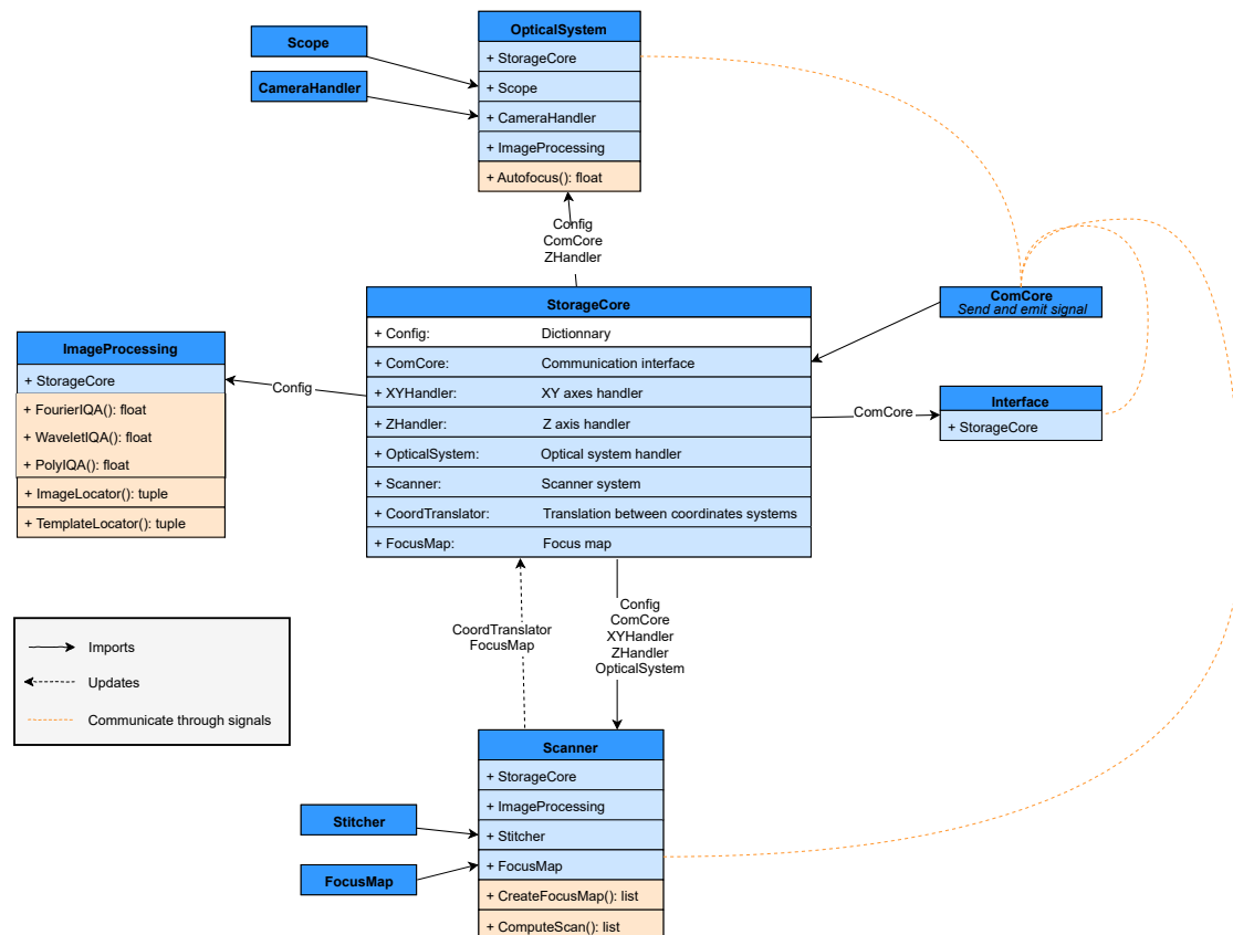
FIGURE 3.11. – Diagramme de classes du logiciel produit et intégrant les recherches exposées dans ce manuscrit, ainsi que leur intégration dans les processus exposé en Section 3.2. Leur fonction est exposée en Section 3.3.3.
