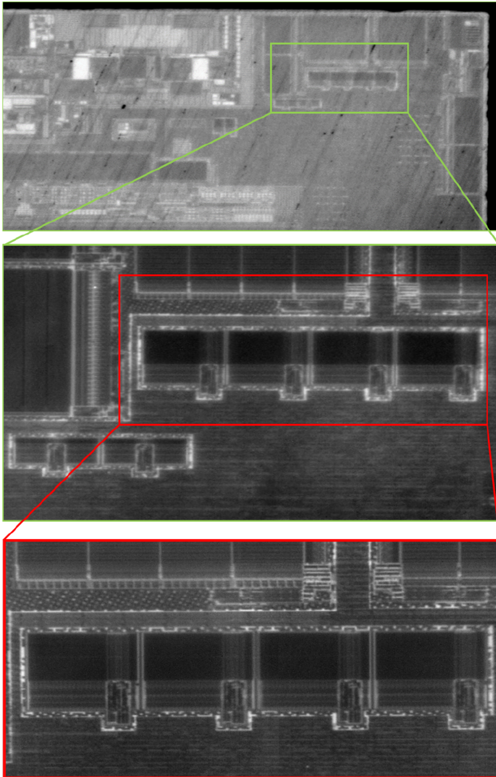
FIGURE 3.4. – Vue multi-résolution d'un circuit intégré, construite à partir de balayages (partiels, pour la démonstration) effectués aux grossissements optiques 5x , 20x et 50x (respectivement de haut en bas).
